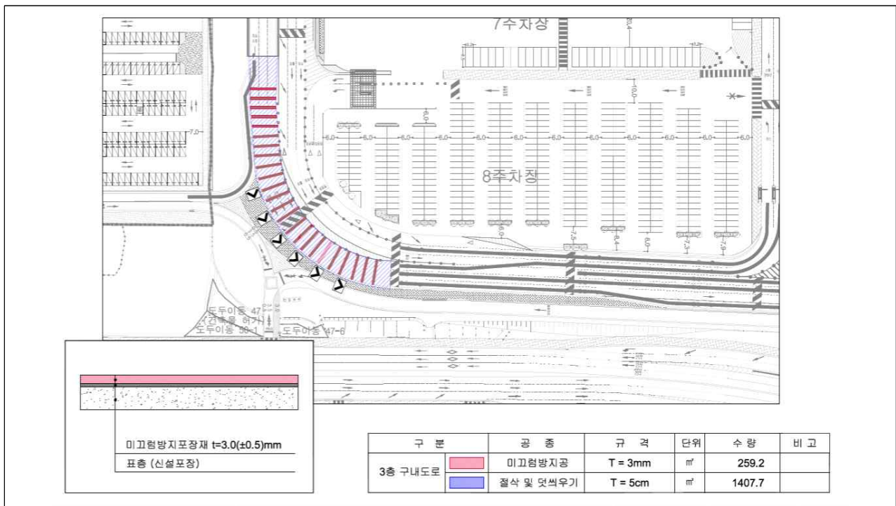
【그림】 아스콘 절삭·덧씌우기 및 미끄럼 방지포장 위치도
