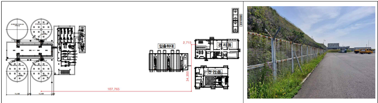
【그림】 탱크 게이징시스템 제어선 지하 매립 구간 (급유 탱크 ~ 관리동)
